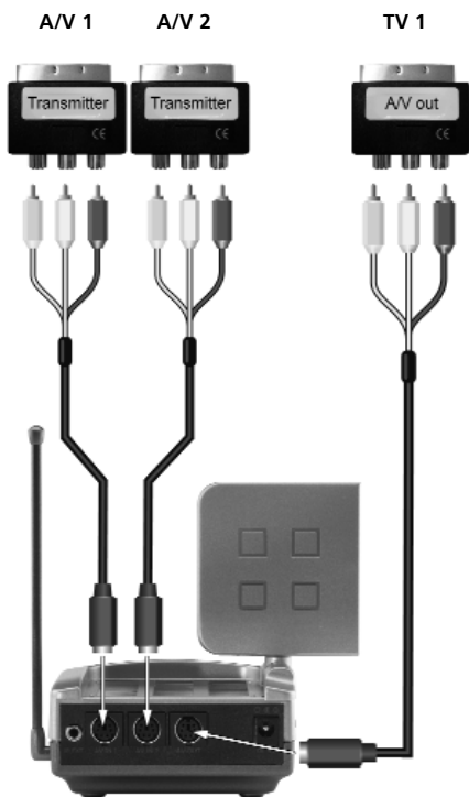
Abbildung 1 A/V SENDER
